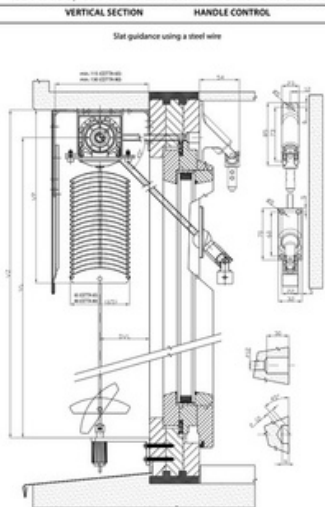
CETTA 80, CETTA 65 EXTERIOR BLIND DIAGRAM
